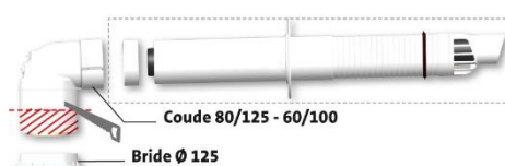
Kit Rolux Renofit® 80/125-60/100
