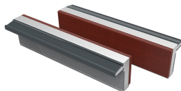
Type F : aluminium + fibre
