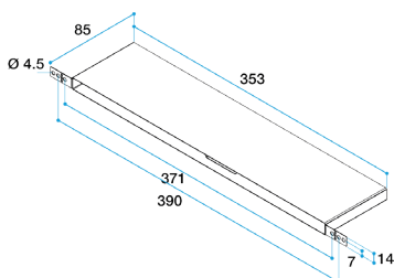
Manchon de raccordement MEA 85
