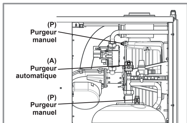
figure 29 - Purgeurs du module hydraulique
