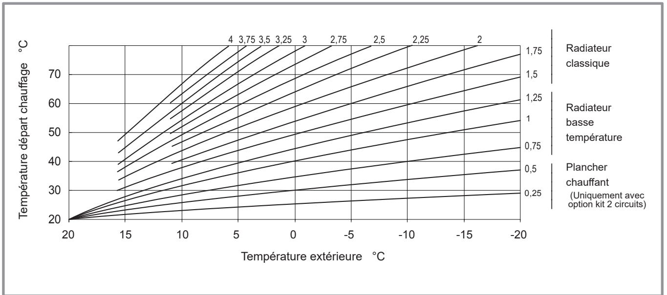
figure 57 - Pente de la courbe de chauffe (ligne 720)
