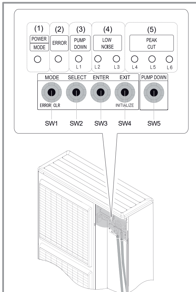
figure 64 - Emplacement des interrupteurs et diodes de l'unité extérieure monophasée
