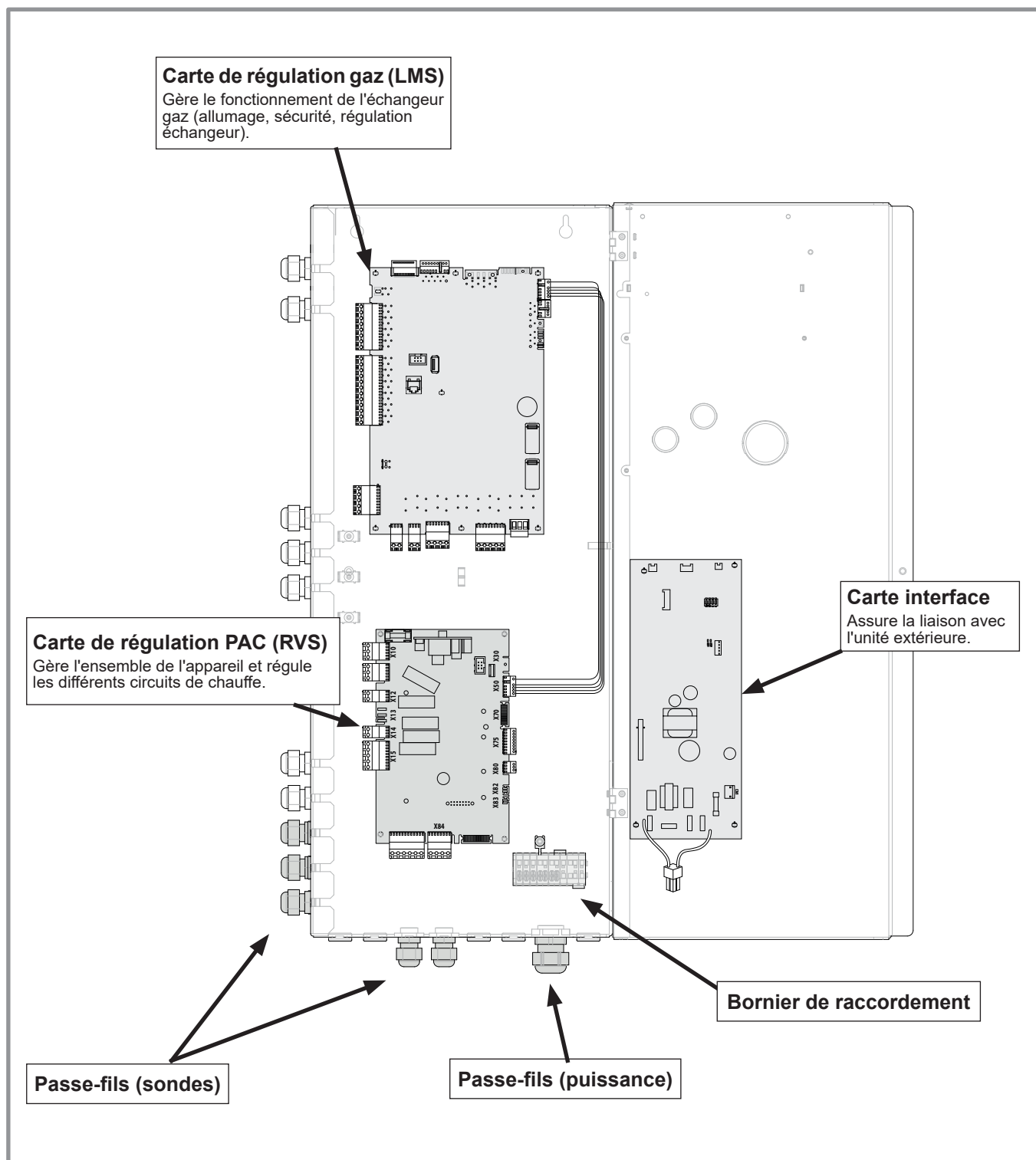
figure 41 - Descriptif du coffret électrique du module hydraulique
