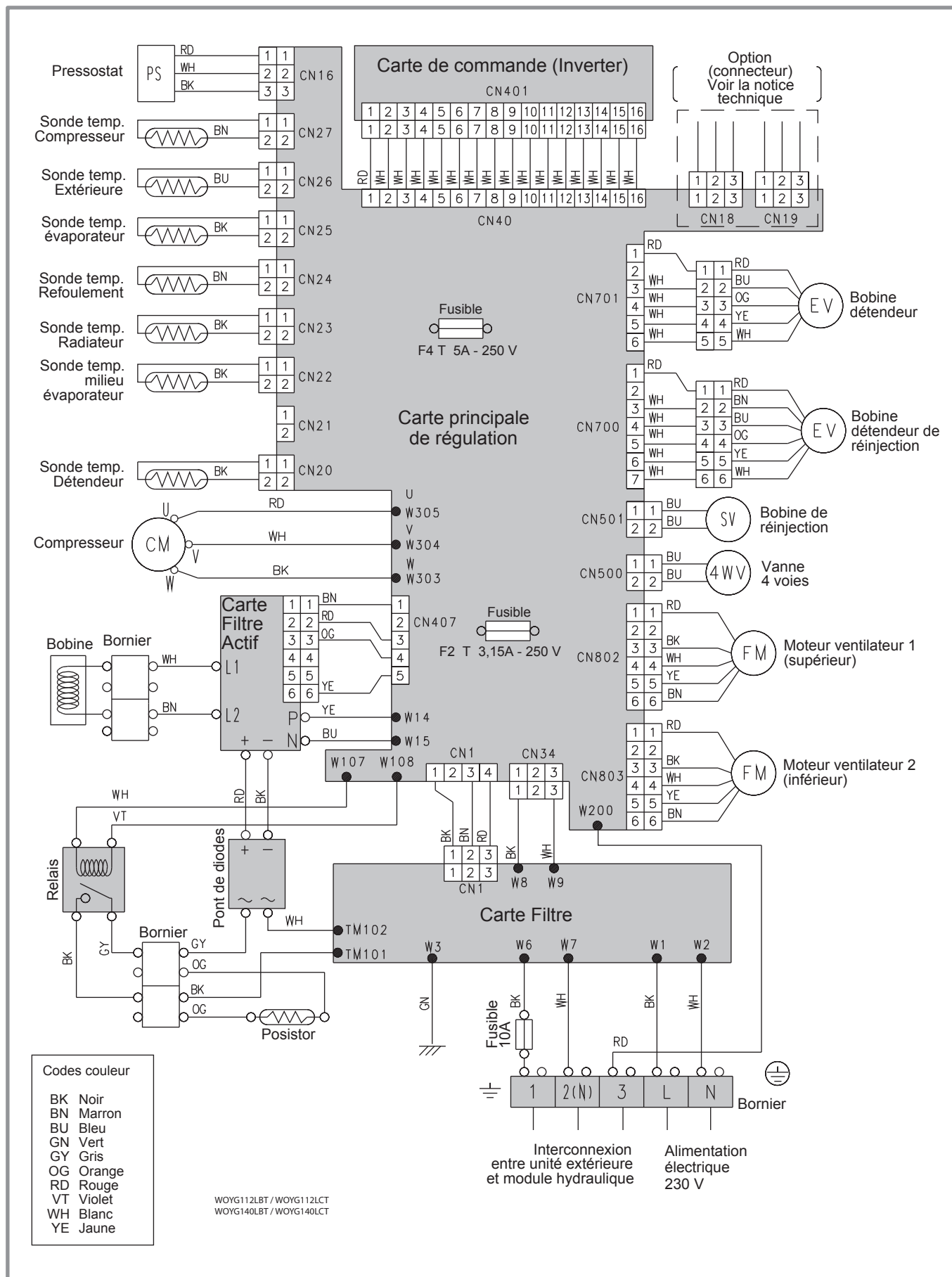
figure 61 - Câblage électrique unité extérieure Modèle alféa hybrid duo gaz monophasée
