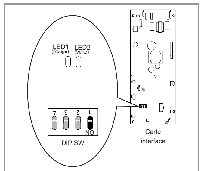
figure 27 - Emplacement des interrupteurs DIP et des diodes sur la carte d'interface du module hydraulique
