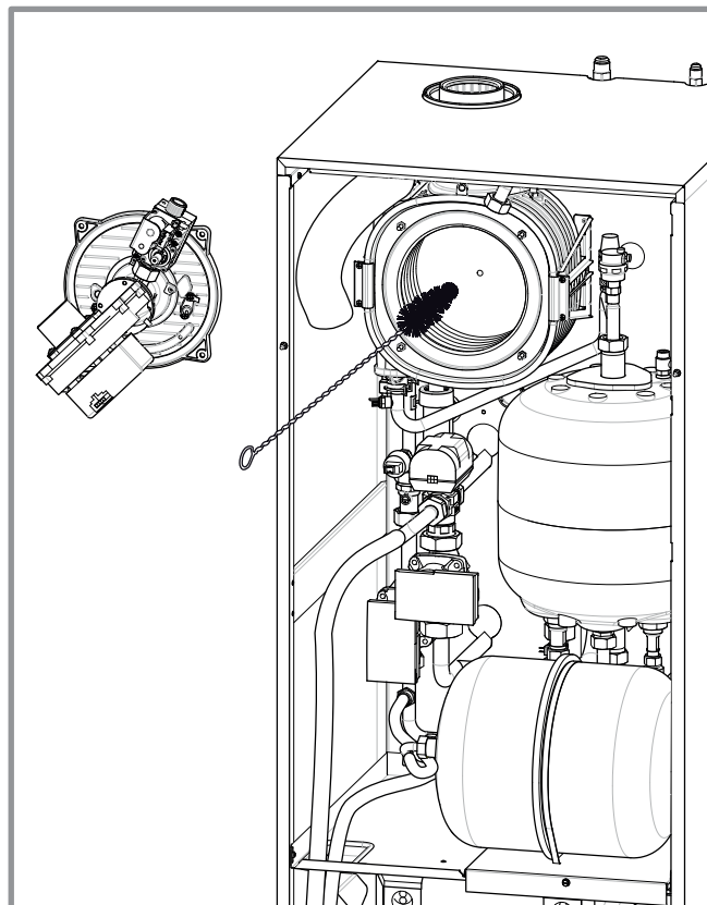
figure 67 - Accès à la chambre de combustion
