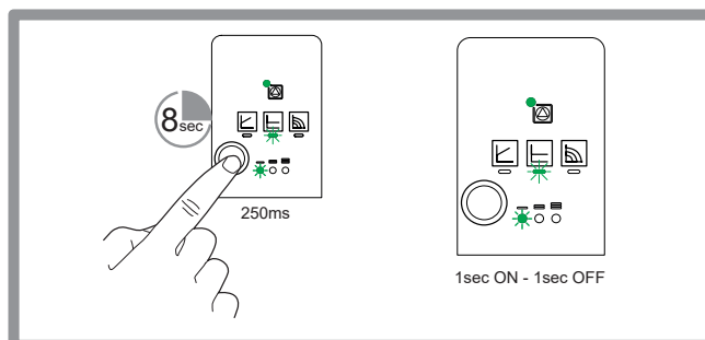
figure 47 - Verrouillage & déverrouillage des réglages du circulateur
