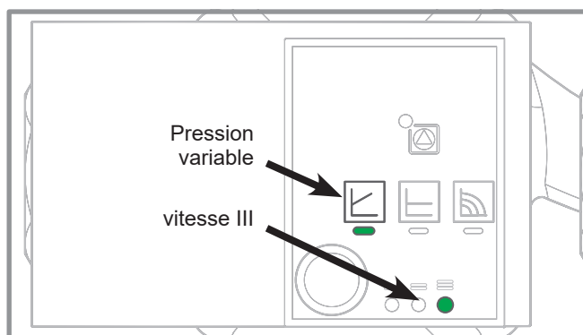
figure 51 - Réglage du circulateur échangeur gaz
