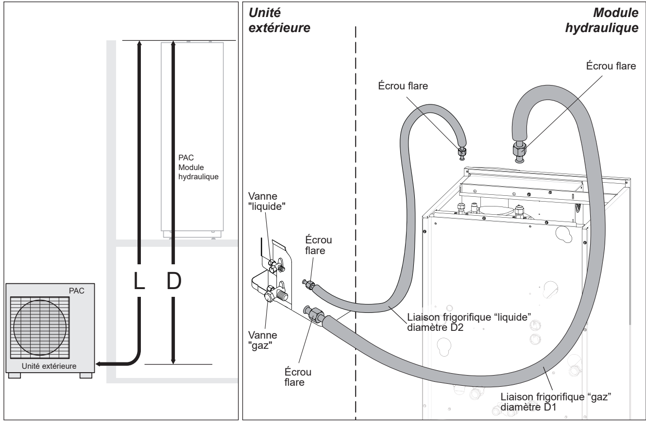
figure 22 - Raccordement des liaisons frigorifiques (diamètres et longueurs permises)
