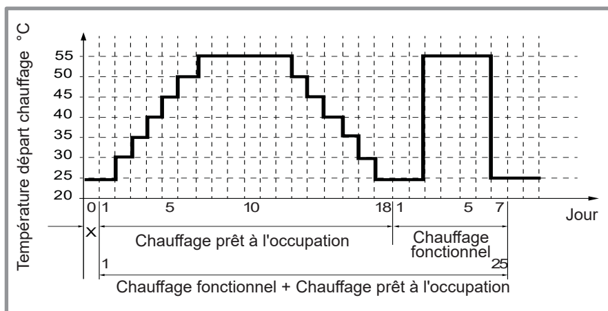
figure 60 - Diagramme des programmes de séchage de dalle
