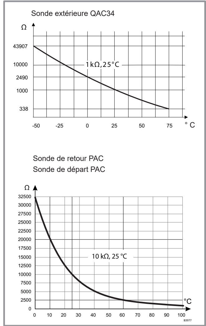
figure 6 - Valeur ohmique des sondes (module hydraulique)
