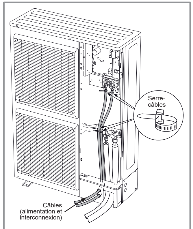
figure 39 - Finalisation de la connexion de l'unité extérieure
