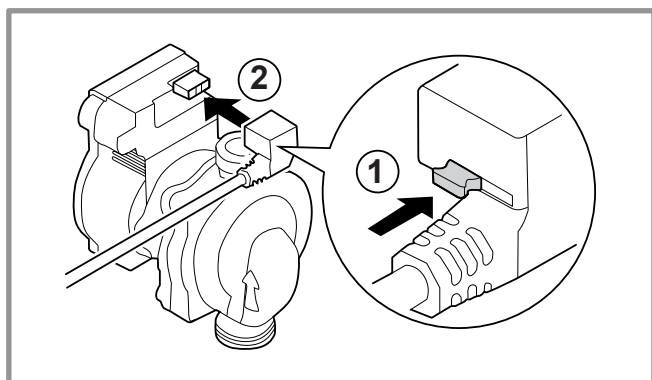
figure 44 - Raccordement du faisceau circulateur
