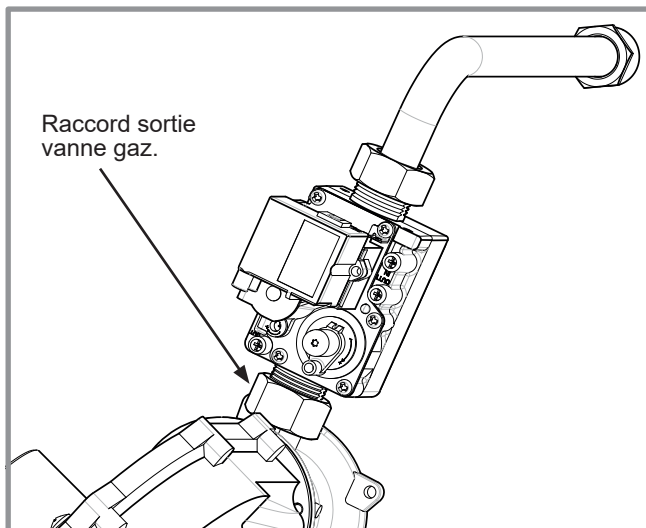
figure 31 - Accès au diaphragme
