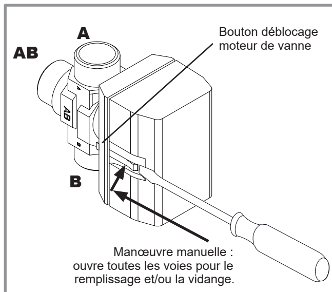
figure 70 - Position intermédiaire de la vanne directionnelle
