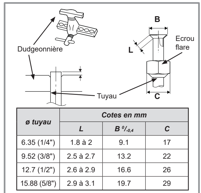
figure 21 - Évasement pour liaisons flare
