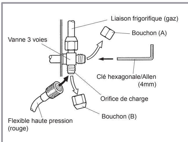
figure 25 - Raccordement du flexible sur la vanne gaz
