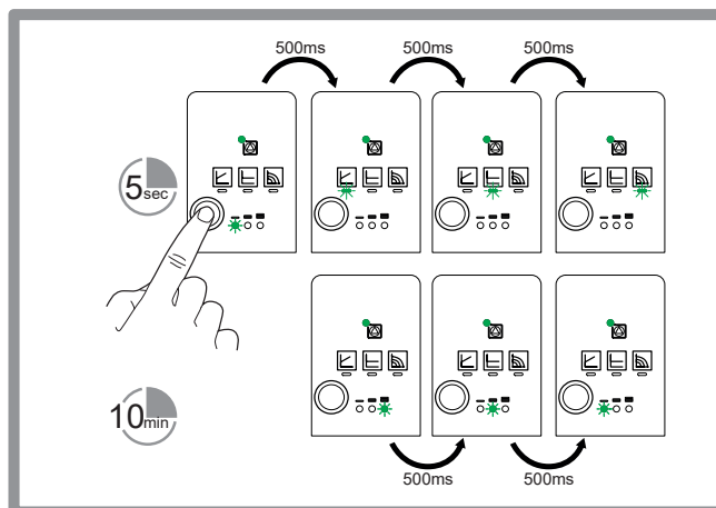
figure 46 - Redémarrage manuel du circulateur
