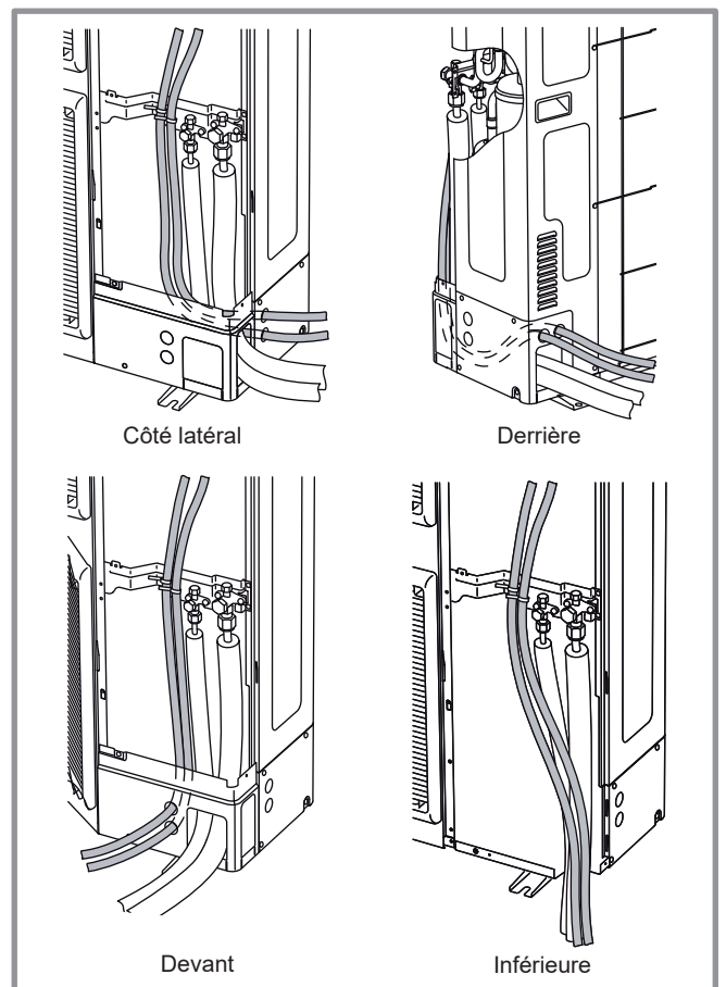
figure 40 - Passages des câbles et liaisons frigorifiques de l'unité extérieure
