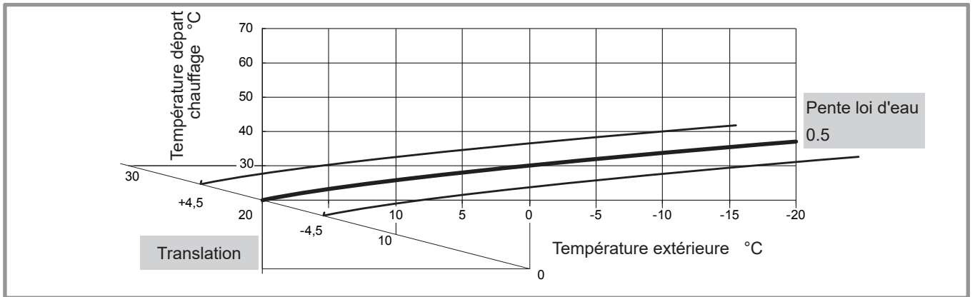
figure 58 - Translation de la courbe de chauffe (ligne 721)
