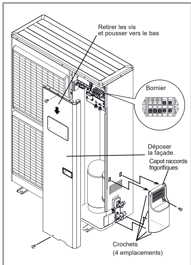
figure 36 - Accès au bornier de l'unité extérieure
