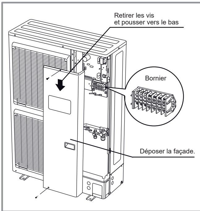
figure 37 - Accès au bornier de l'unité extérieure
