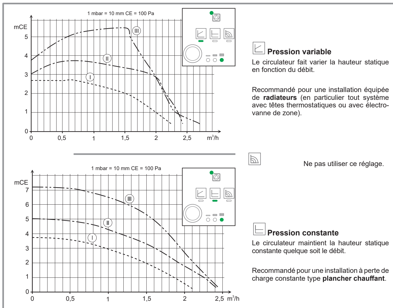
figure 50 - Pressions et débits hydrauliques disponibles
