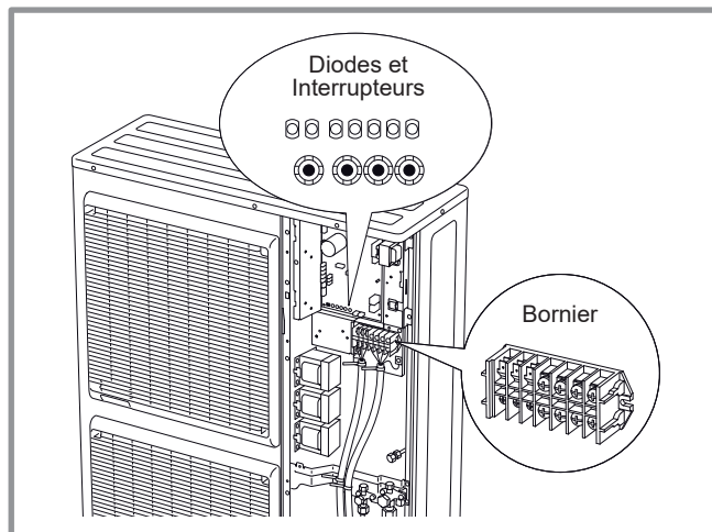
figure 65 - Emplacement des interrupteurs et diodes de l'unité extérieure.
