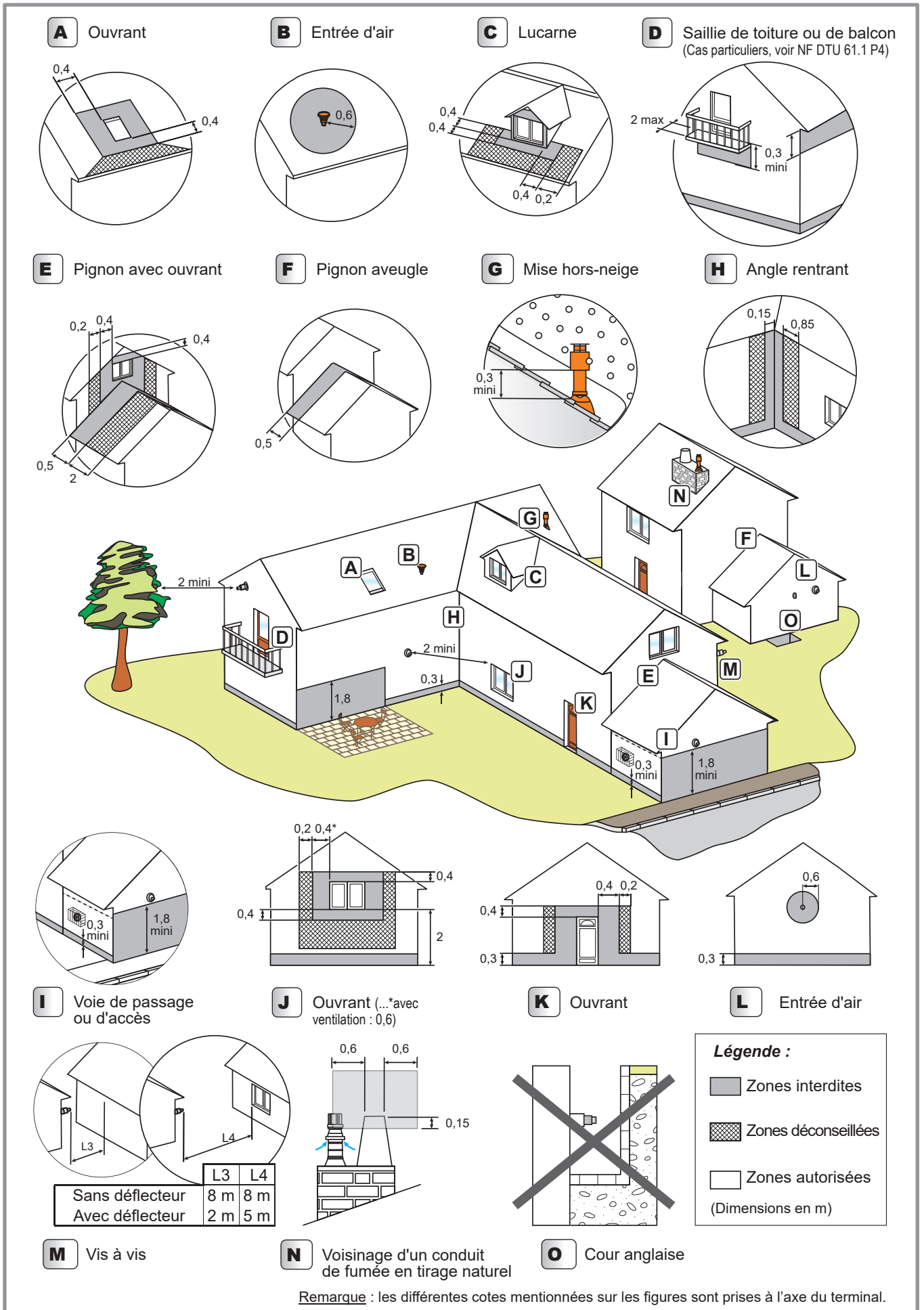
figure 20 - Règles d'implantation du terminal pour chaudières gaz étanches (C13, C33, C53)
