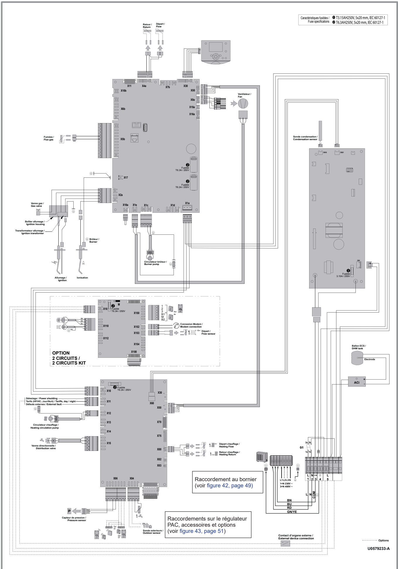
figure 63 - Câblage électrique module hydraulique (hors raccords installateur)
