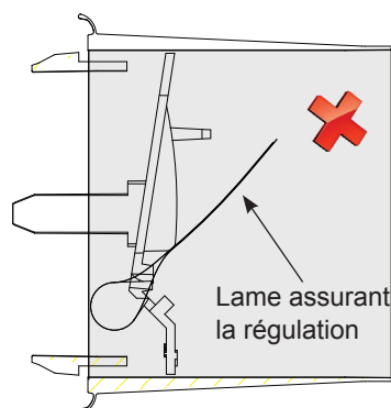
Mauvaise position (Vue en coupe)
