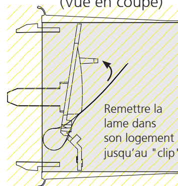
Si mauvaise position, remettre en position la lame (Vue en coupe)
