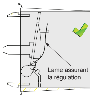
Bonne position (Vue en coupe)
