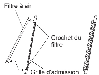
Grille d'admission
