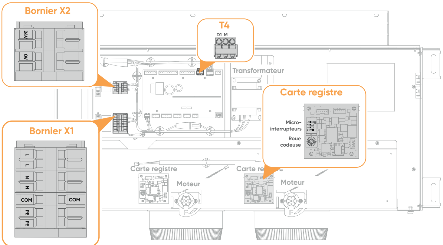
Coffret électrique du Shogun 1.1
