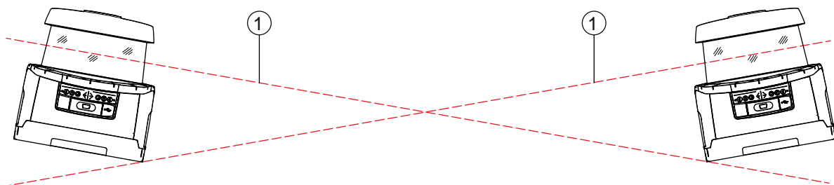
Fig. 7.10: Montage côte à côté, sans décalage en hauteur, alignement croisé
