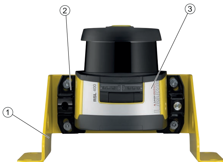
Fig. 7.4: Exemple : montage sur une arête chanfreinée
