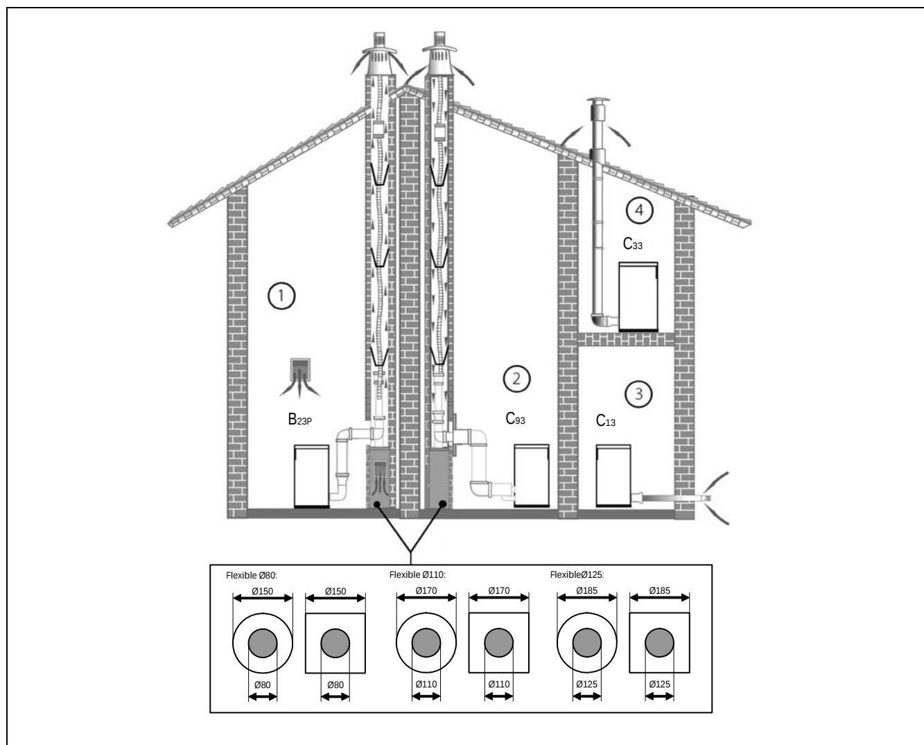
Configurations conduits condensation fioul
